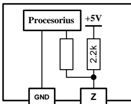
Įėjimo ekvivalentinė schema
